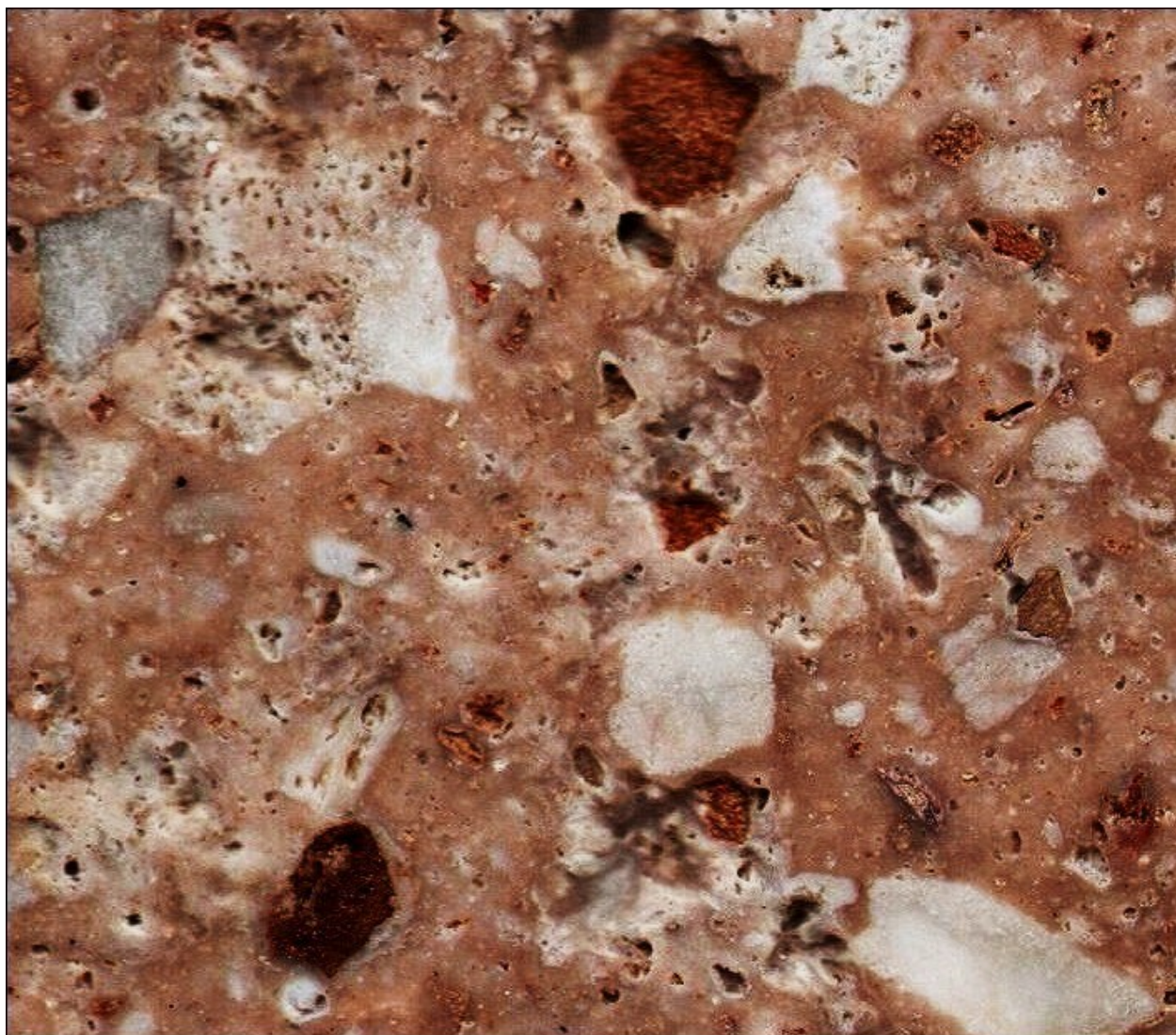
Abb. 17: Burgruine Tierberg, Mörtelstück, Mörtel geschliffen (Abstand der rotbraunen Tonschieferstücke: 17 mm), farblich überhöht. Foto (2023).
